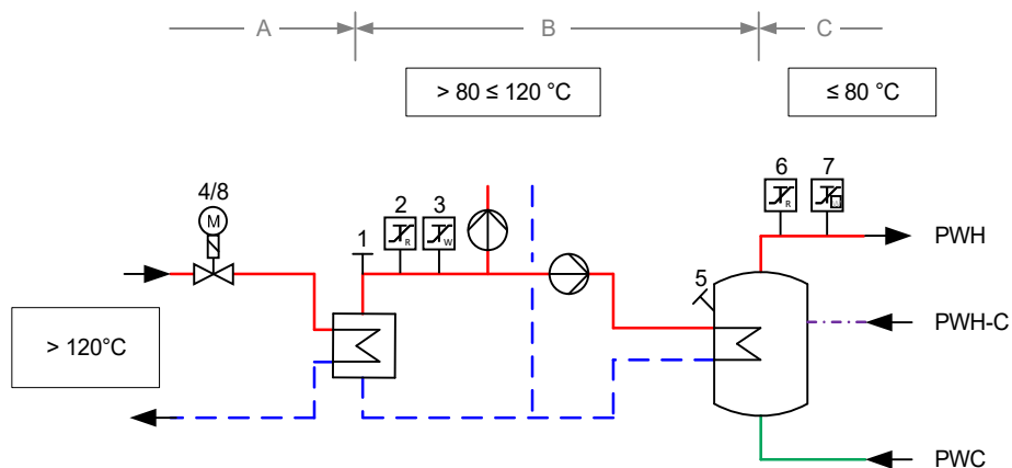
Abbildung zur Tabelle 7: Erforderliche sicherheitstechnische Ausrüstung nach Zeile 2/3
