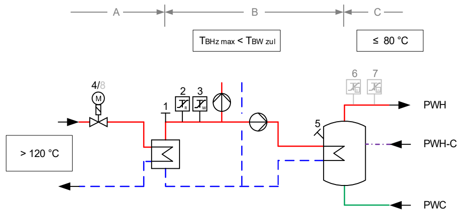
Abbildung zur Tabelle 7: Erforderliche sicherheitstechnische Ausrüstung nach Zeile 1; grau dargestellte Komponenten nicht erforderlich
