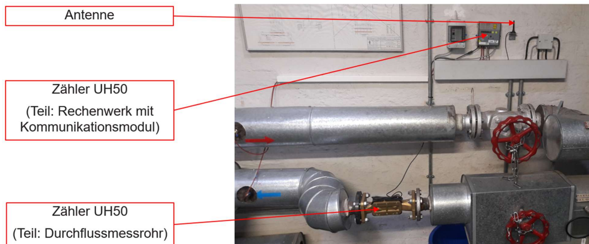
Abbildung 2: Installation Zählerfernauslesung (Beispielbild)
