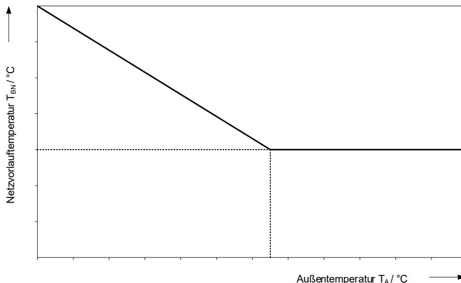
Abbildung 1: Netzhaupttemperatur T_{BN} in Abhängigkeit von der Außentemperatur T_A ; prinzipieller Verlauf einer gleitend-konstanten Fahrweise
