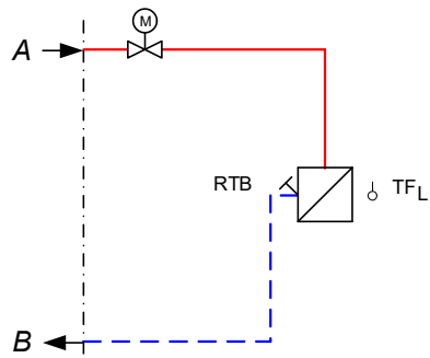
Abbildung 8: Hauszentrale-Raumluftheizung Prinzipschaltbilder für den indirekten Anschluss
