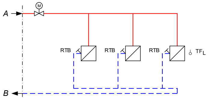
Abbildung 8: Hauszentrale-Raumluftheizung Prinzipschaltbilder für den indirekten Anschluss
